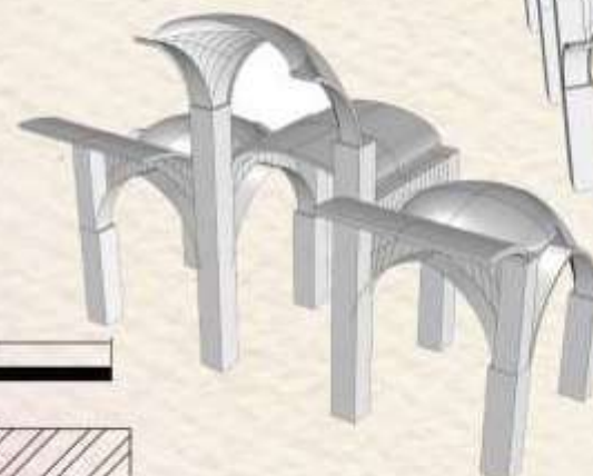
پرسپکتیو برش B Section B
