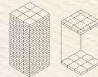
آجرچینی تقاطع دیوار ۶۰ با ۶۰
