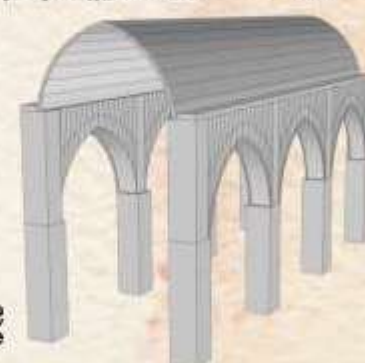
طاق آهنگ روی تویزه باربر
