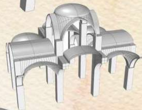
پرسپکتیو برش A Section A
